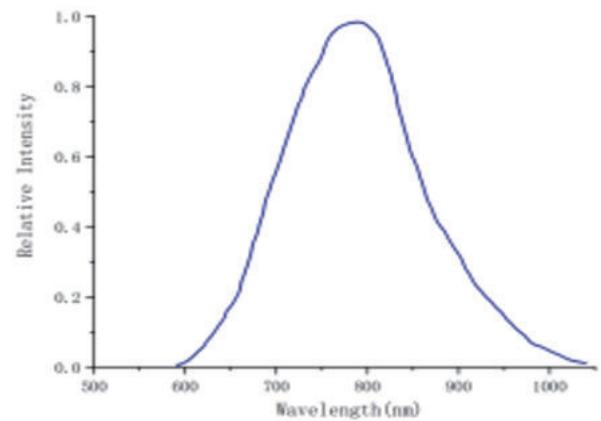
钛宝石发射光谱
