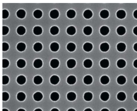
400nm 周期四方排布
