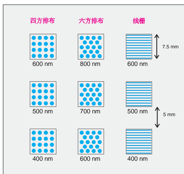
MHSL400-800 各图案布局示意图
