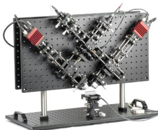
光片显微系统
