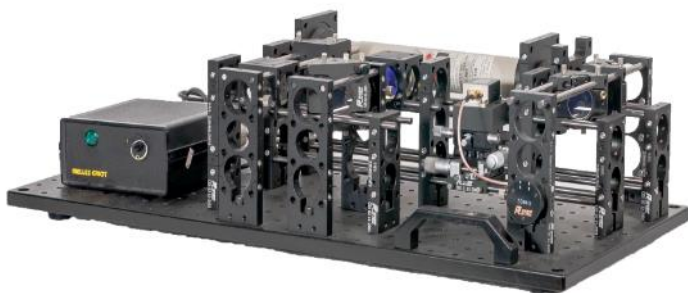
外差干涉系统
