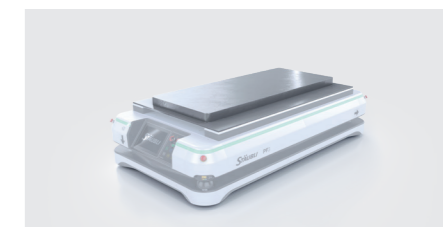
顶升单元(行程 +100mm) + 美式托盘适配器 高: 465 mm
